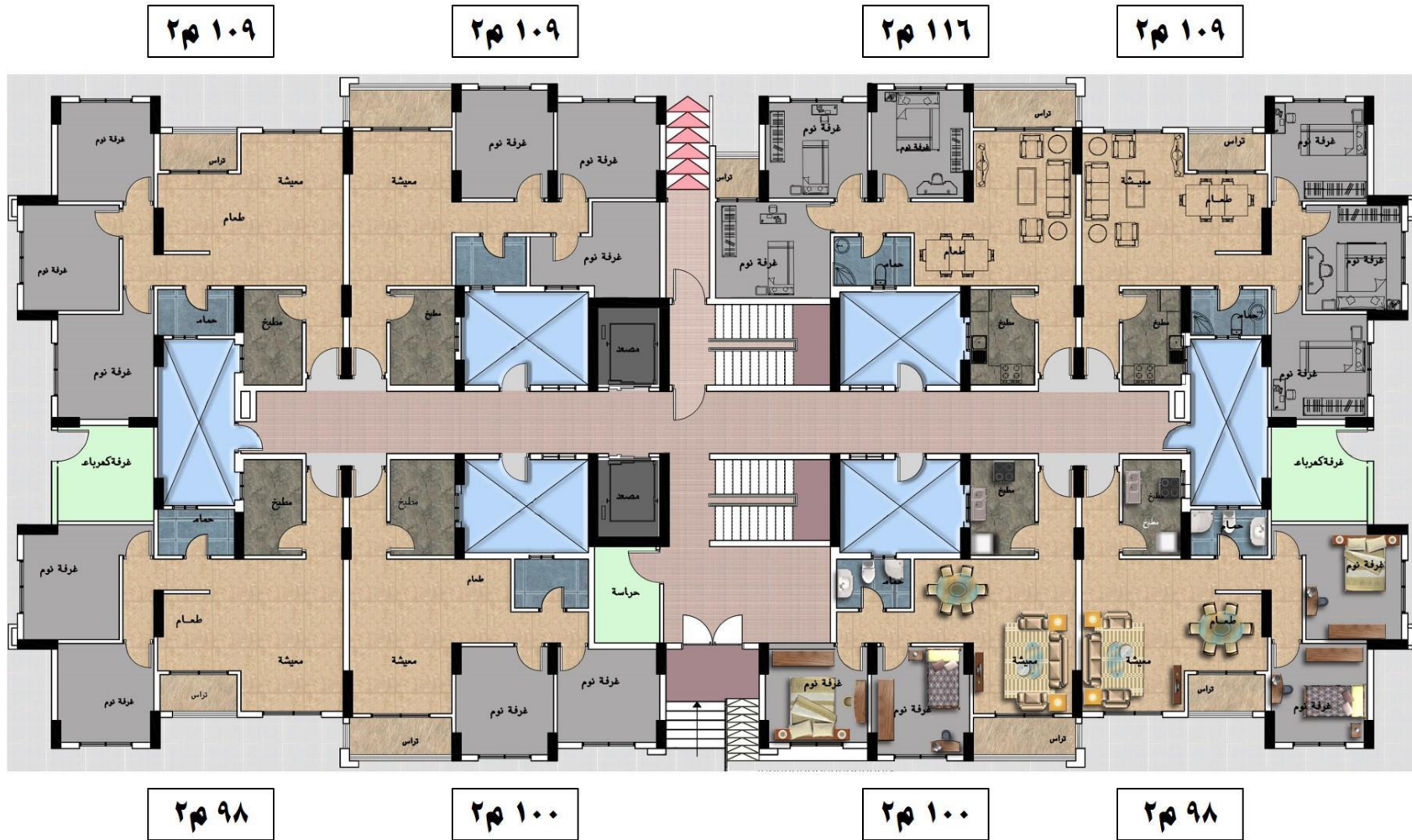
المسقط الأفقي للدور الأرضي
